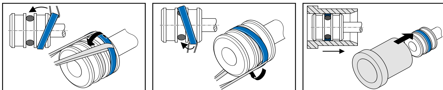
2. Fitting with mounting tape and calibration sleeve | Montage avec du ruban adhésif et un manchon d'étalonnage | Instalación con cinta de montaje y la manga de calibración | Instalação com fita de montagem e manga de calibração
